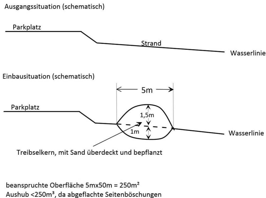
Abb. 12: Aufbau einer Treibseldüne am Beispiel Noer
