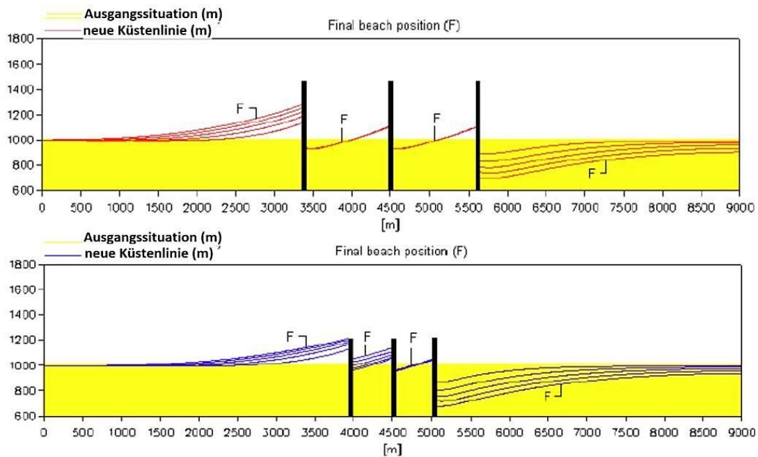
Abb. 8: Bühnenfeld mit unterschiedlich langen Bühnen und Abstand (verändert nach MANGOR et. al 2017)
