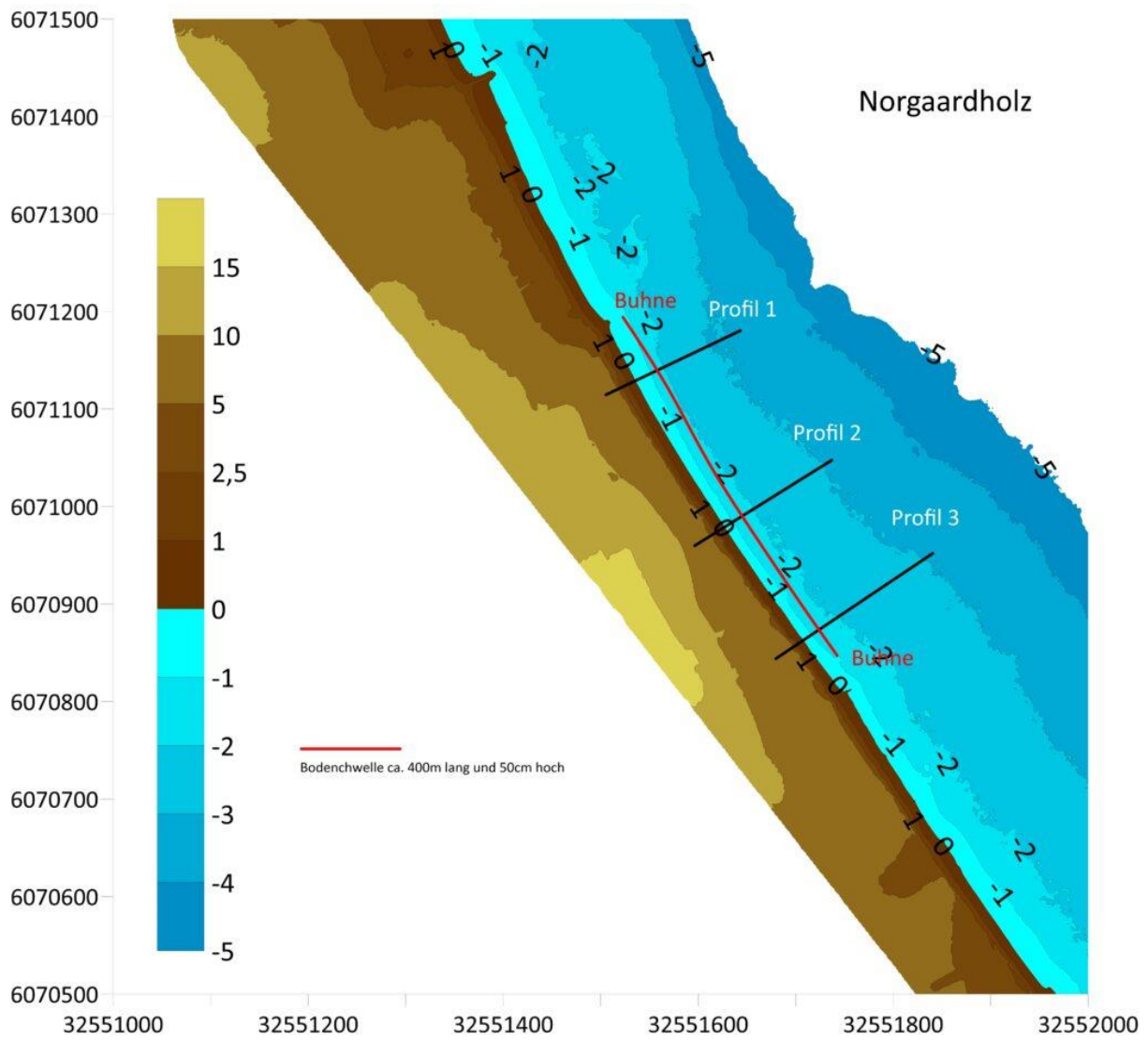
Abb. 14a: Draufsicht Bodenschwellen
