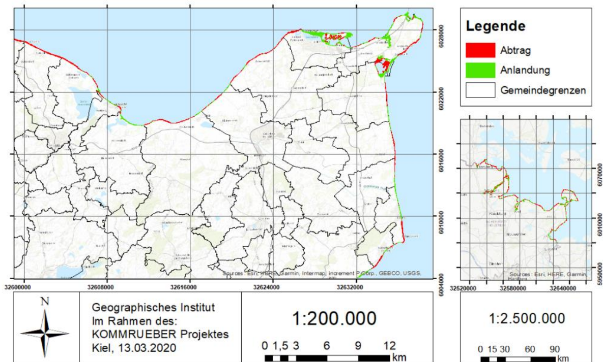
Abb. 3: Die Veränderung der Uferlinie von 1878 bis 2010 am Beispiel Eckernförder Bucht und Ostholstein (nach Landesbetrieb für Küstenschutz, Nationalpark und Meeresschutz Schleswig-Holstein, LKN-SH 2017)
