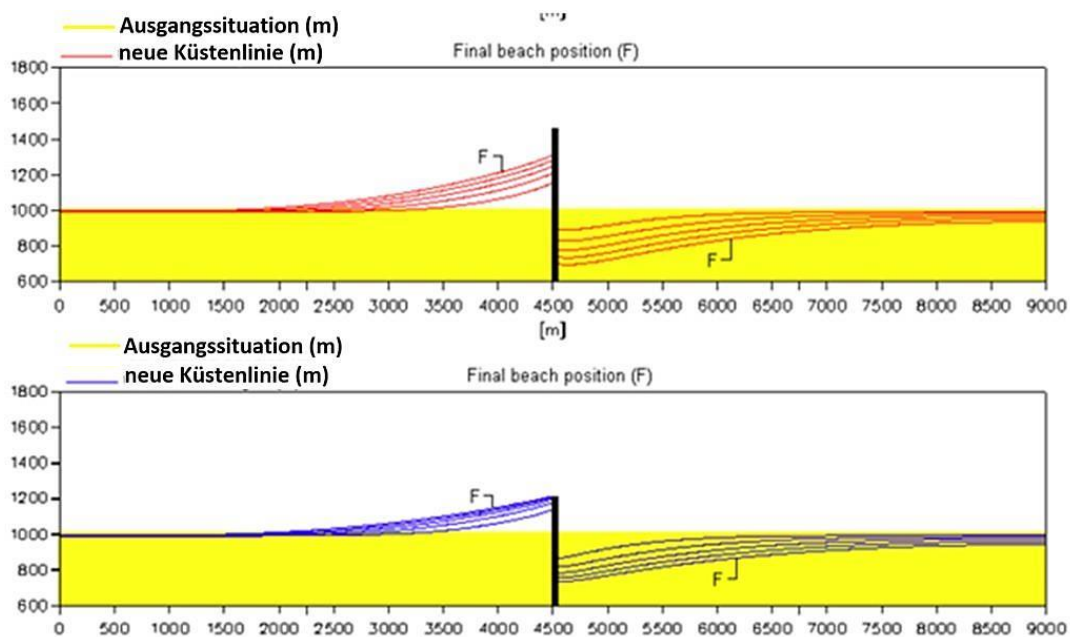
Abb. 7: Einzelbuhnen mit unterschiedlicher Länge (verändert nach MANGOR et. al 2017)
